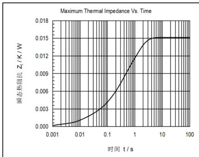
图2. 瞬态热阻曲线及分析曲线
